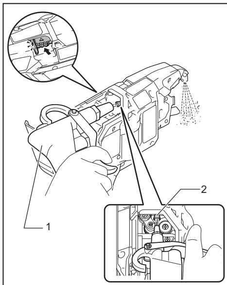
► 1. Pistola sacudidora de polvo 2. Guía
