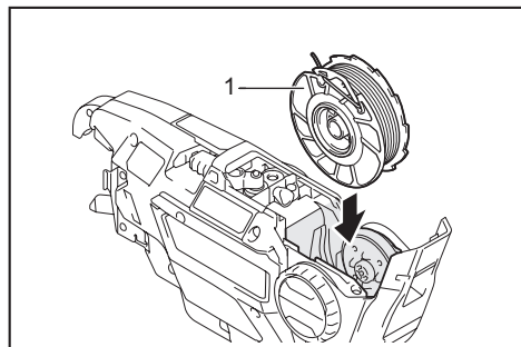
► 1. Carrete de alambre
