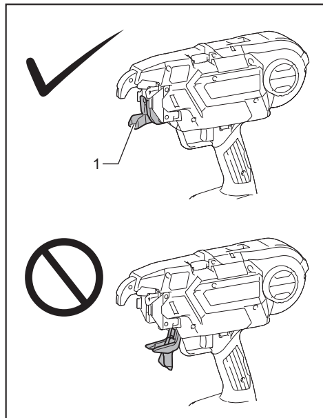
► 1. Guía de rizo
