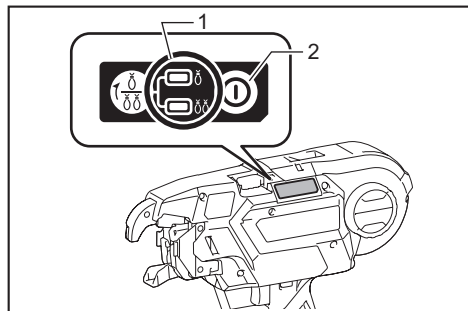
► 1. Lámpara de modo de amarre 2. Botón de alimentación
